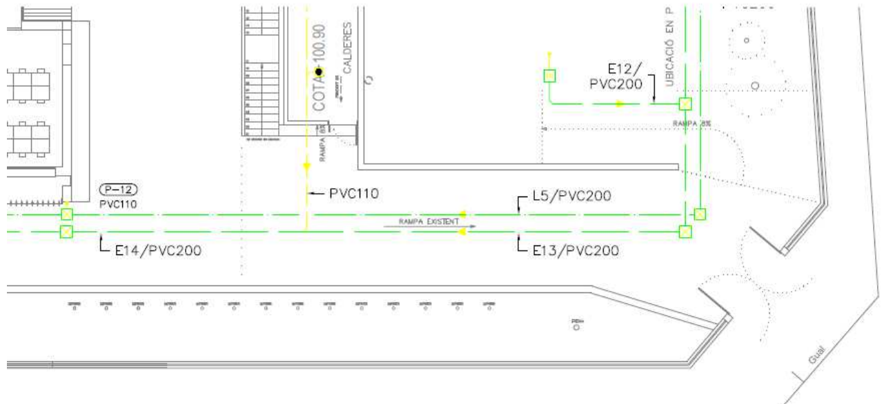
Plànol d'emplaçament
