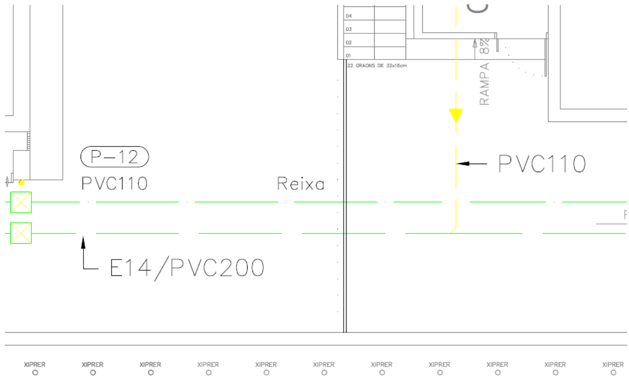
Plànol de situació de la reixa recollectora
